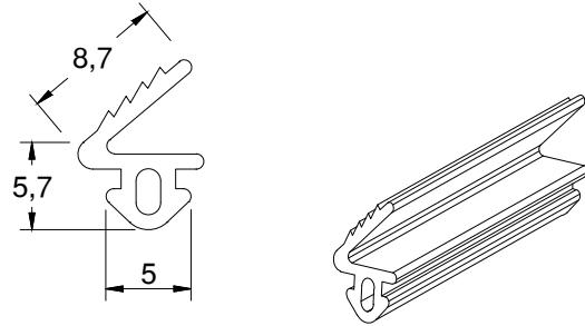
GUA-239 - Guarnição p/ marco EPDM
