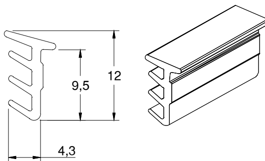
GUA-259 - Guarnição do vidro
