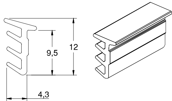
GUA-259 - Guarnição do vidro EPDM
