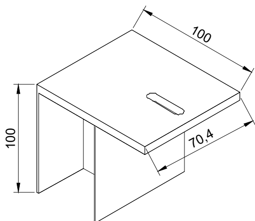
ANC-965 - Ancoragem telescópica para coluna FC-202
