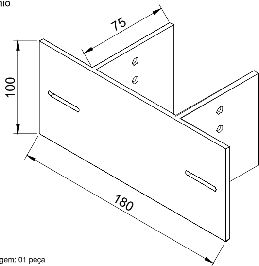
ANC-951 - Ancoragem para coluna
