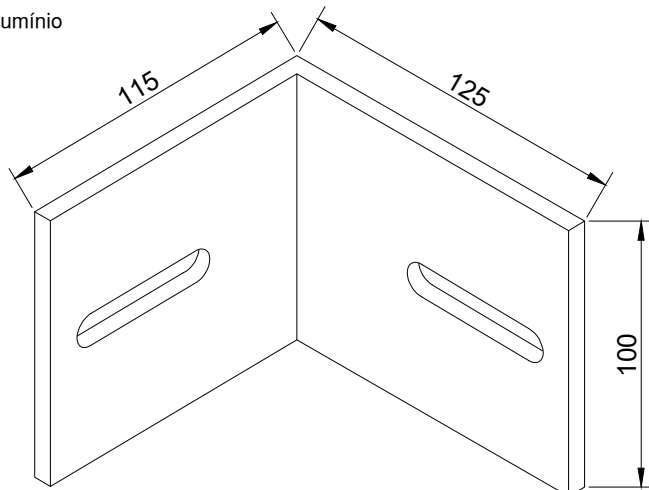
ANC-967 - Ancoragem da coluna 90°
