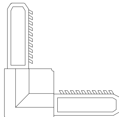
CNX-08 - Cantoneira de conexão p/ tela mosquiteira
